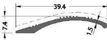
CODE / KOD 20-130-00 THEORETICAL WEIGHT kg/m TEORİK AĞIRLIK kg/m 0.183
