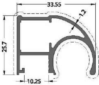
CODE / KOD 21-152-00 THEORETICAL WEIGHTkg/m TEORİK AĞIRLIK kg/m 0.437
