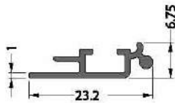
CODE / KOD 21-137-010 THEORETICAL WEIGHTkg/m TEORİK AĞIRLIK kg/m 0.121
