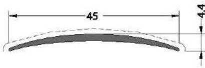
CODE / KOD 20-149-00 THEORETICAL WEIGHT kg/m TEORİK AĞIRLIK kg/m 0.171
