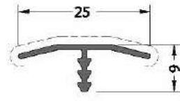
CODE / KOD 20-102-00 THEORETICAL WEIGHT kg/m TEORİK AĞIRLIK kg/m 0.103
