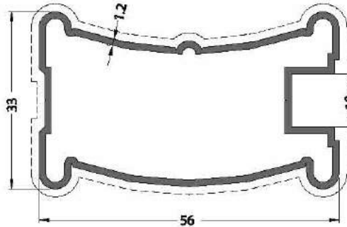
CODE / KOD 21-166-012 THEORETICAL WEIGHTkg/m TEORİK AĞIRLIK kg/m 0.659
