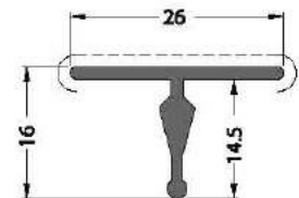
CODE / KOD 21-160-00 THEORETICAL WEIGHTkg/m TEORİK AĞIRLIK kg/m 0.191
