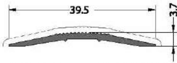
CODE / KOD 20-124-00 THEORETICAL WEIGHT kg/m TEORİK AĞIRLIK kg/m 0.157
