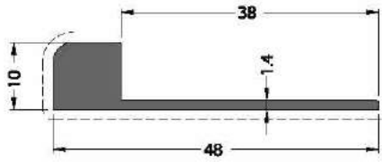
CODE / KOD 21-180-00 THEORETICAL WEIGHT kg/m TEORİK AĞIRLIK kg/m 0.410
