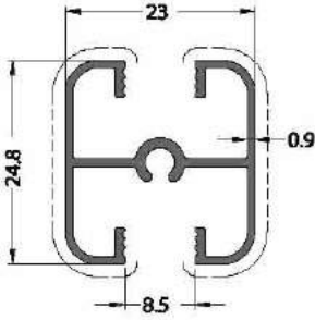
CODE / KOD THEORETICAL 21-210-00 WEIGHTkg/m TEORİK AĞIRLIK kg/m 0.291
