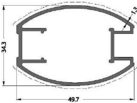
CODE / KOD 21-159-013 THEORETICAL WEIGHTkg/m TEORİK AĞIRLIK kg/m 0.632
