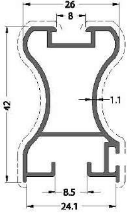
CODE / KOD 21-125-011 THEORETICAL WEIGHT kg/m TEORİK AĞIRLIK kg/m 0.498
