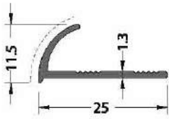
CODE / KOD 20-145-00 THEORETICAL WEIGHT kg/m TEORİK AĞIRLIK kg/m 0.158
