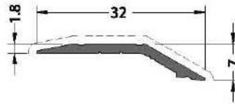
CODE / KOD 20-150-00 THEORETICAL WEIGHT kg/m TEORİK AĞIRLIK kg/m 0.142
