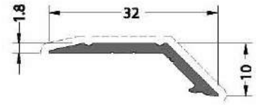
CODE / KOD 20-151-00 THEORETICAL WEIGHT kg/m TEORİK AĞIRLIK kg/m 0.159
