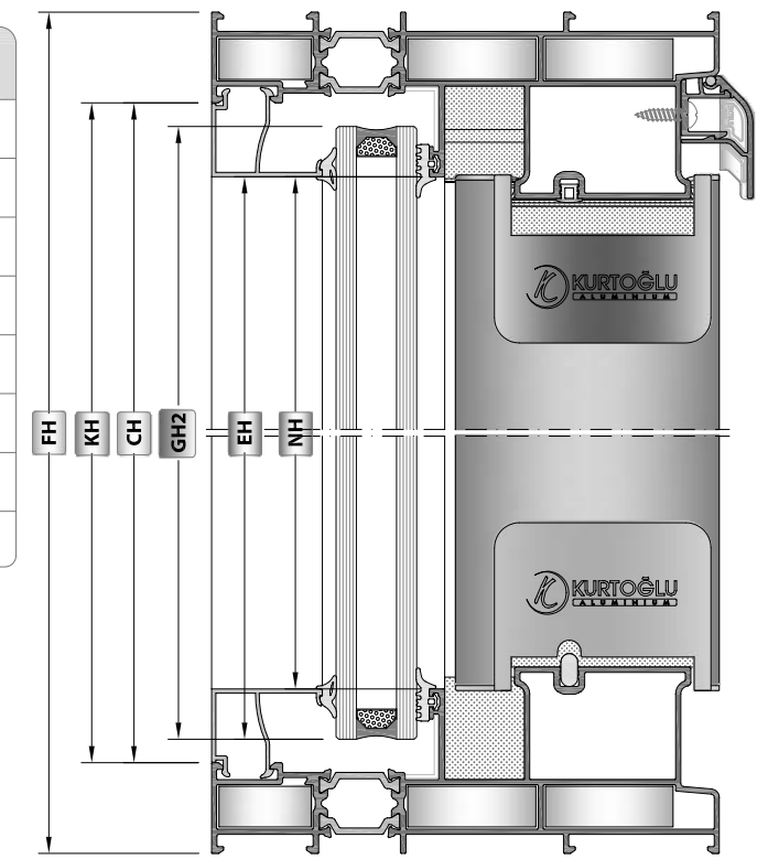
A-A SECTION / A-A KESİTİ
